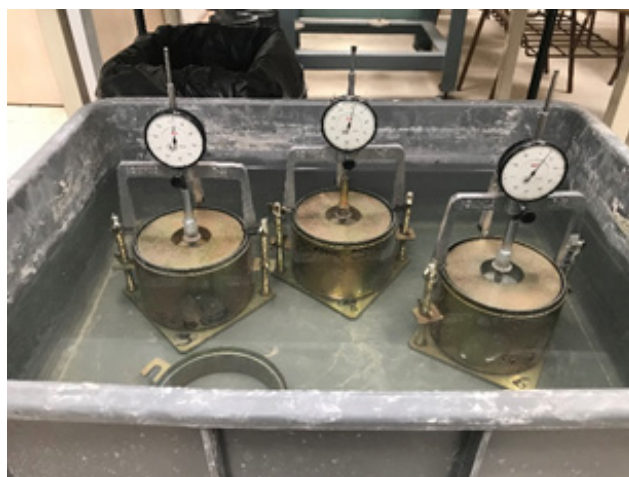
Ensayos CBR con inmersión.
